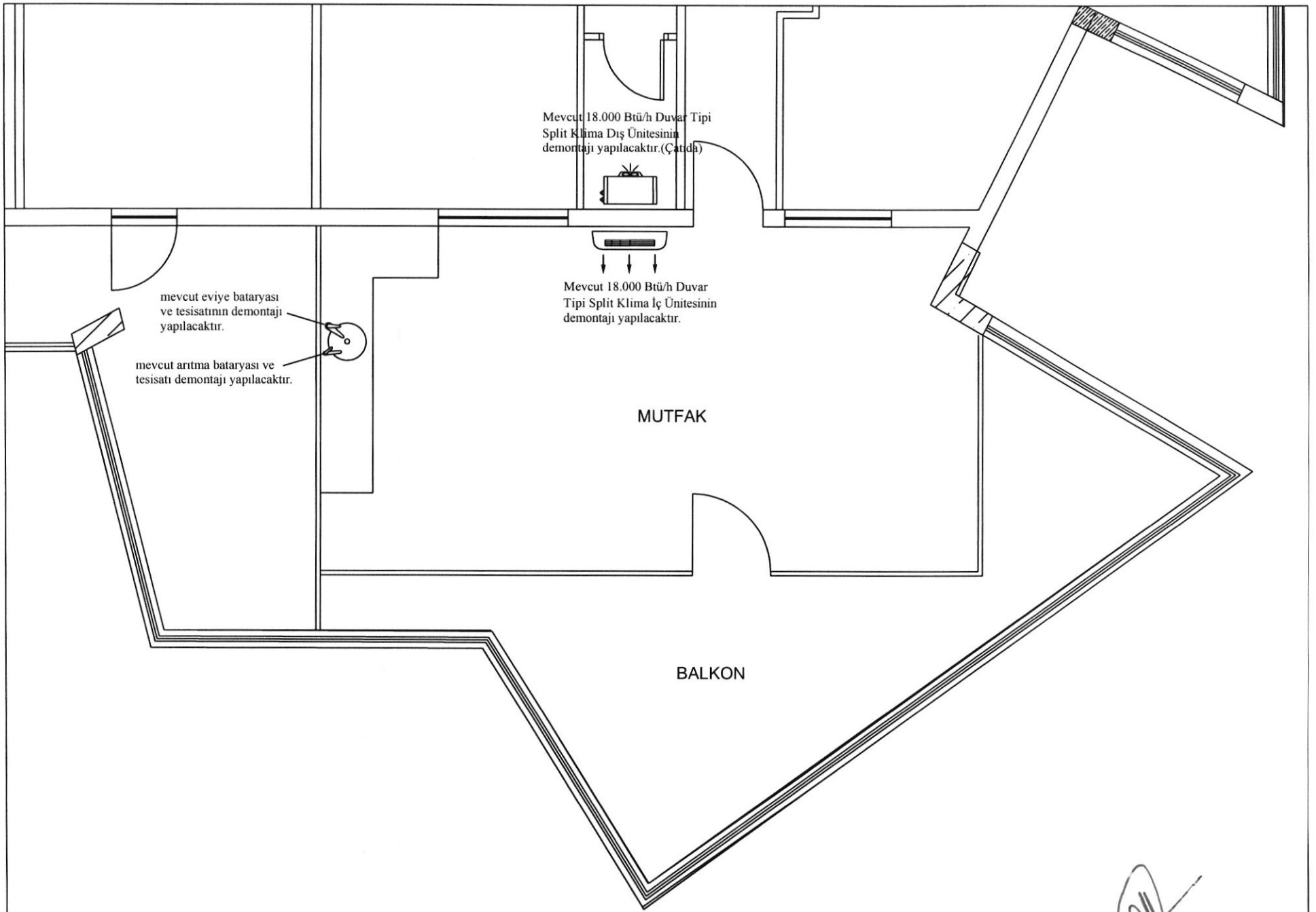
BİLGİ İŞLEM DAİRE BAŞKANLIĞI TERAS 2 MEKANİK TESİSAT MEVCUT PLAN
